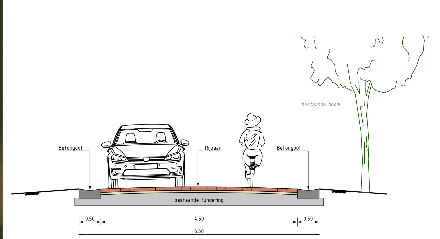
PRINCIEPROFIEL RIJBAAN Schaal 1:50
