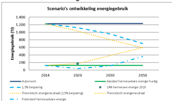
figuur 2.1 Scenario's ontwikkeling energiegebruik
