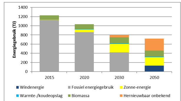
figuur 2.2 Ontwikkeling hernieuwbare energieopwekking
