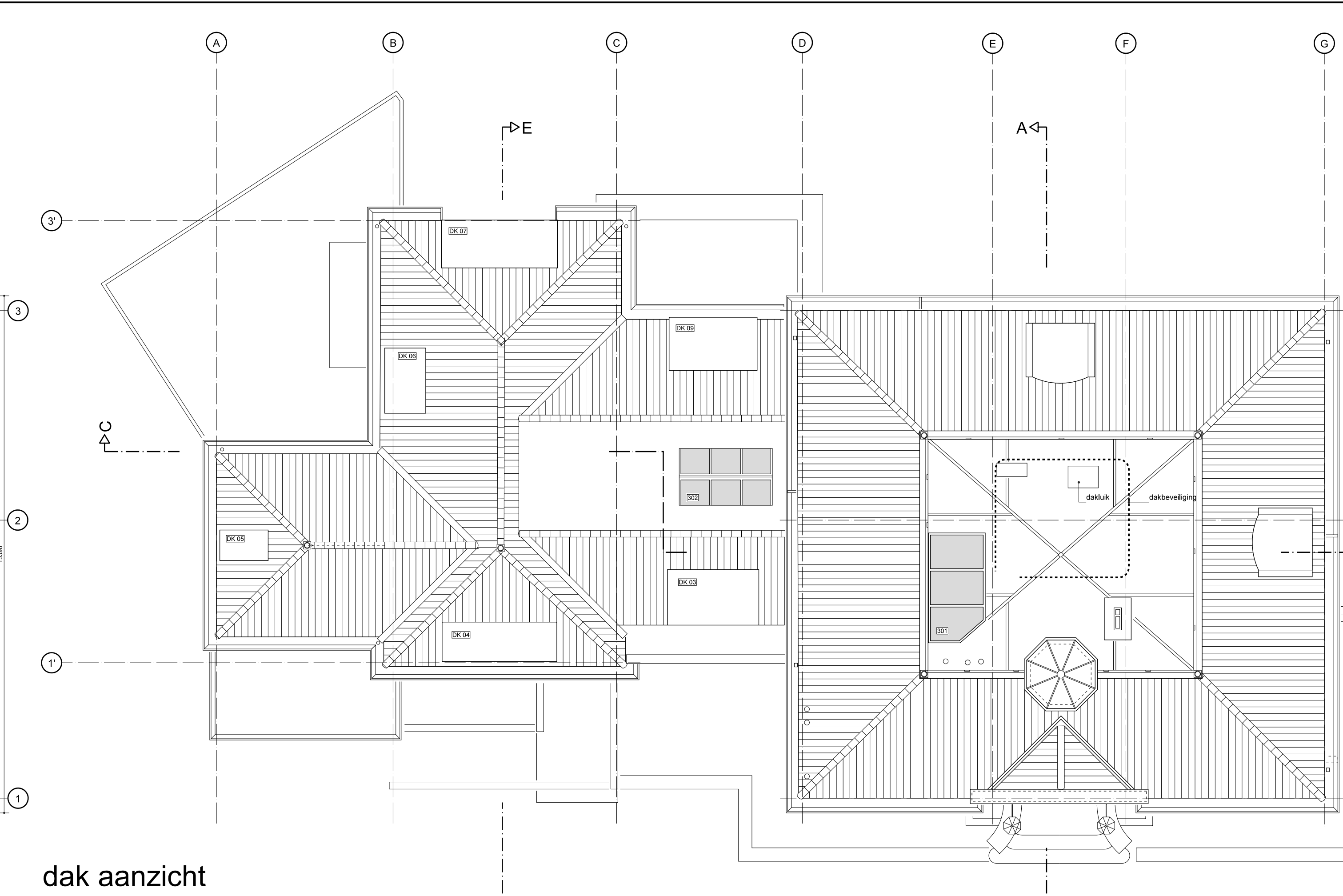
dak aanzicht
