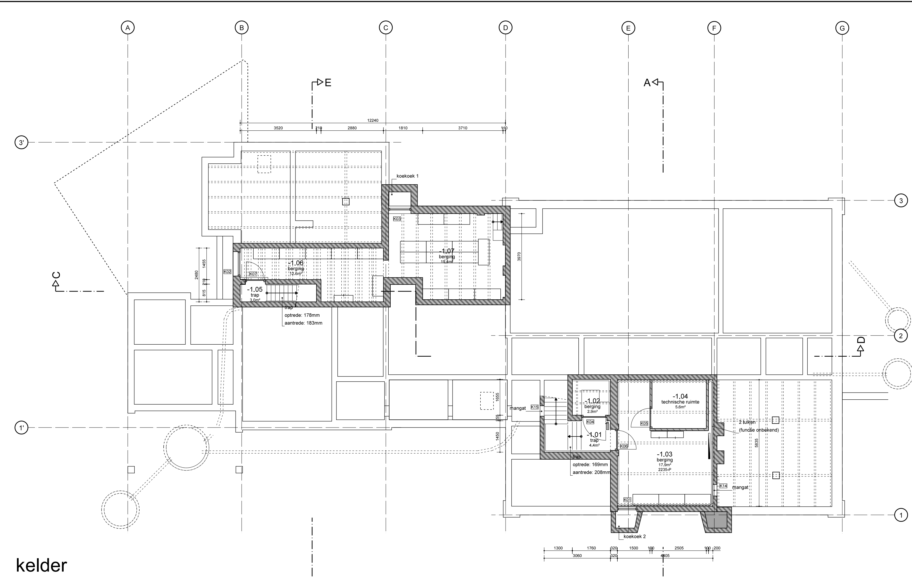
kelder
