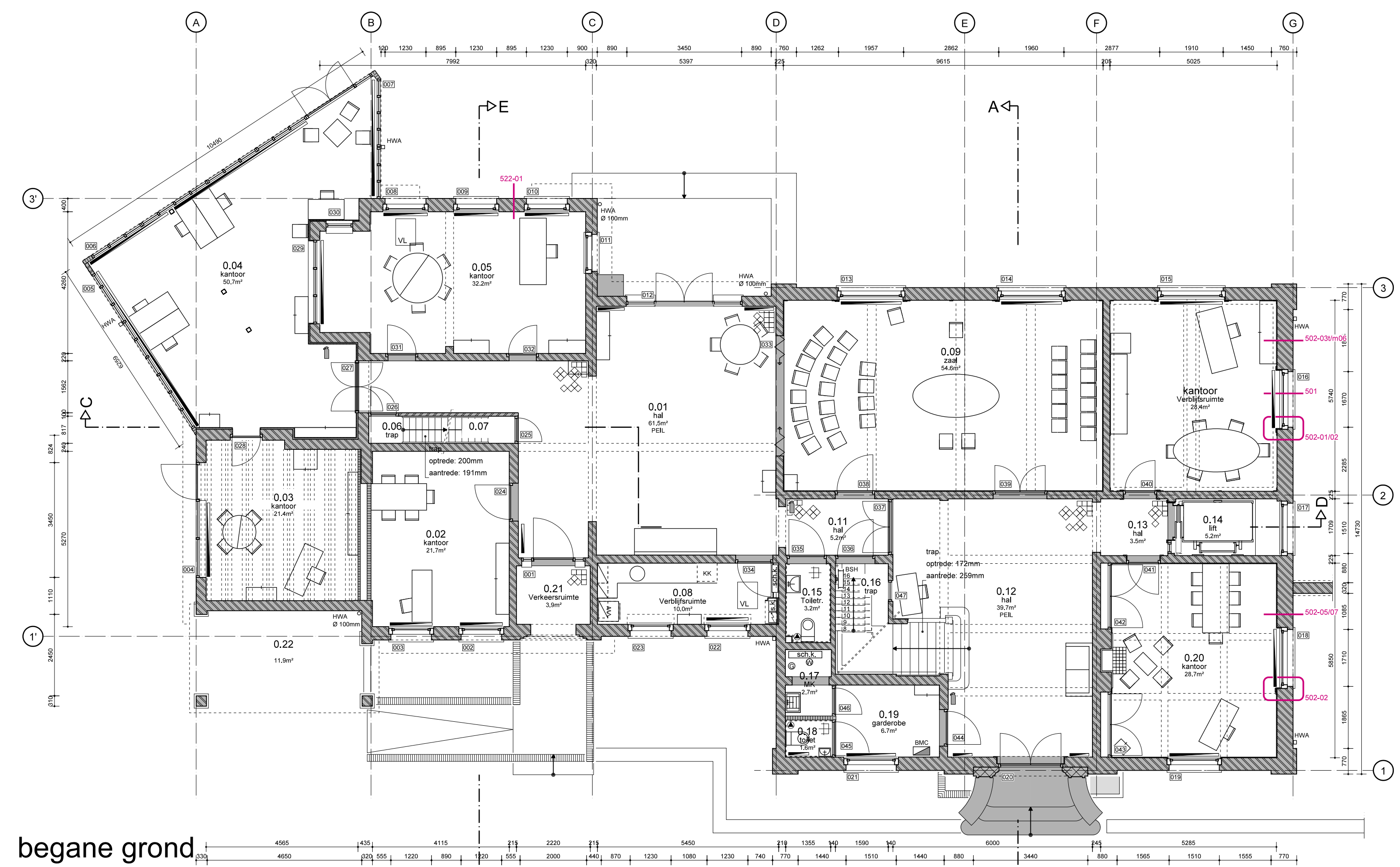
begane grond
